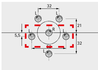
Рис. 17 Карта сверления
