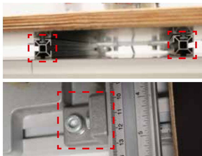
Рис. 8: Каркас с центрирующими шпонками
