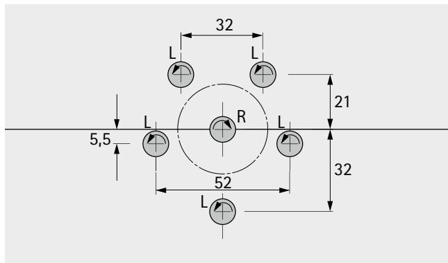
Рис. 10: Карта сверления
