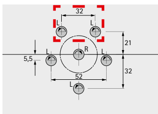
Рис. 20: Карта сверления
