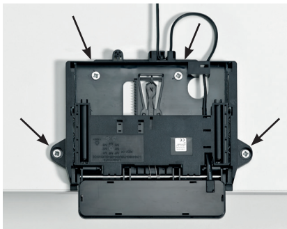
Abb. 30: Schraublöcher für die Montage des Handschalters LegaData Drive Touch Comfort.
