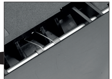
Abb. 36: Ende der Feder in Nase unter dem Schlitten eingehakt
