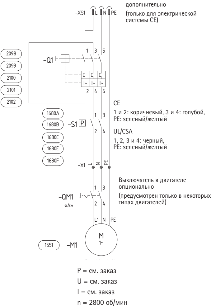
BlueMax Mini 1 фазы
